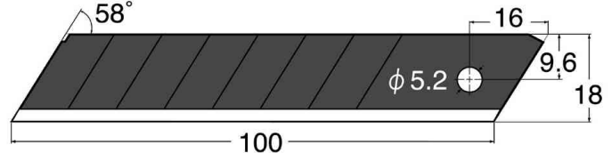
Detailansicht Ersatzklingen BL13P
