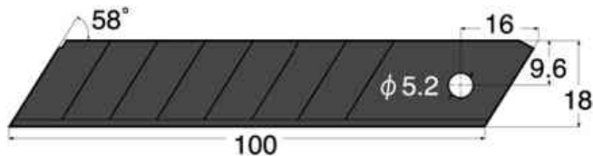
Detailansicht Ersatzklingen BL-51P
