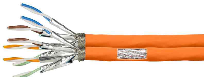
Symbolbild: Installationskabel Kat. 7, S/FTP - 1.000 MHz, Duplex
