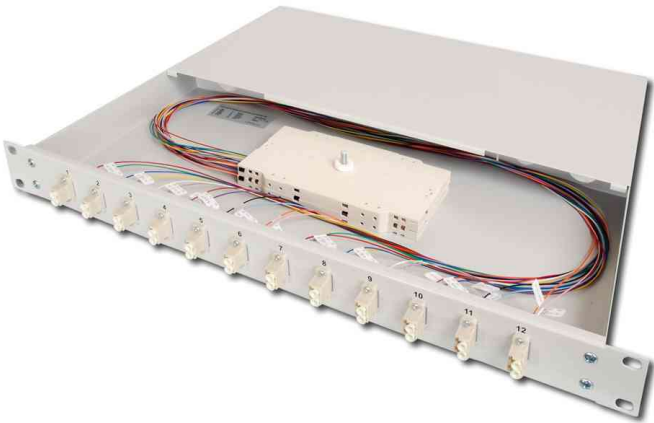
19" Glasfaser LWL Spleißbox, 12 x LC
